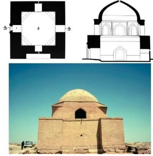
Görsel 7.20. Aslan Cazip Türbesi Planı ve Görünüşü
