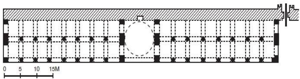
Görsel 7.17. Leşker-i Bazar Ulu Camii Planı
