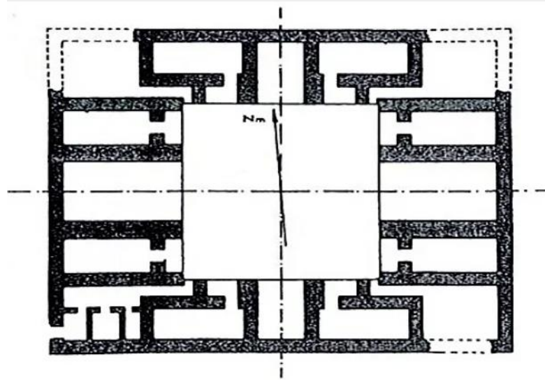
Görsel 7.25. Rey Medresesi Planı
